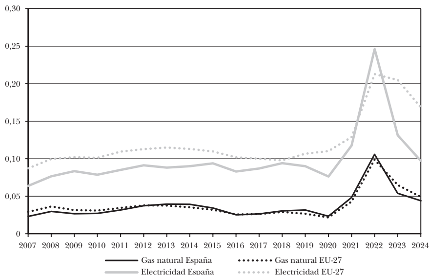
GRÁFICO 2.18: Evolución del coste de la energía. España y EU-27, 2007-2024 (€/kWh)
